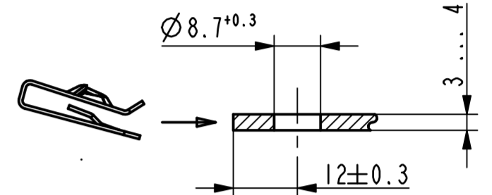
Einbausituation / assembly situation 1:1
