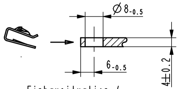
Einbausituation / assembly situation 1:1
